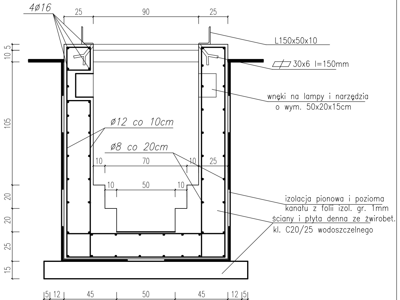
PRZEKRÓJ PIONOWY I-I
